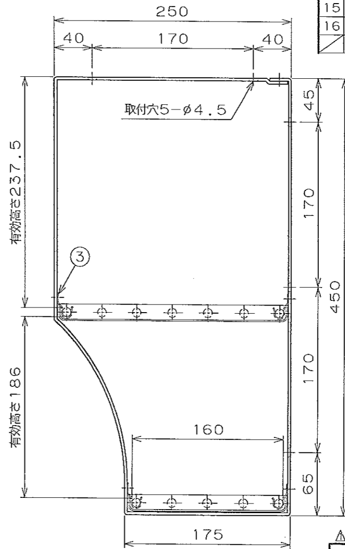
側面図
