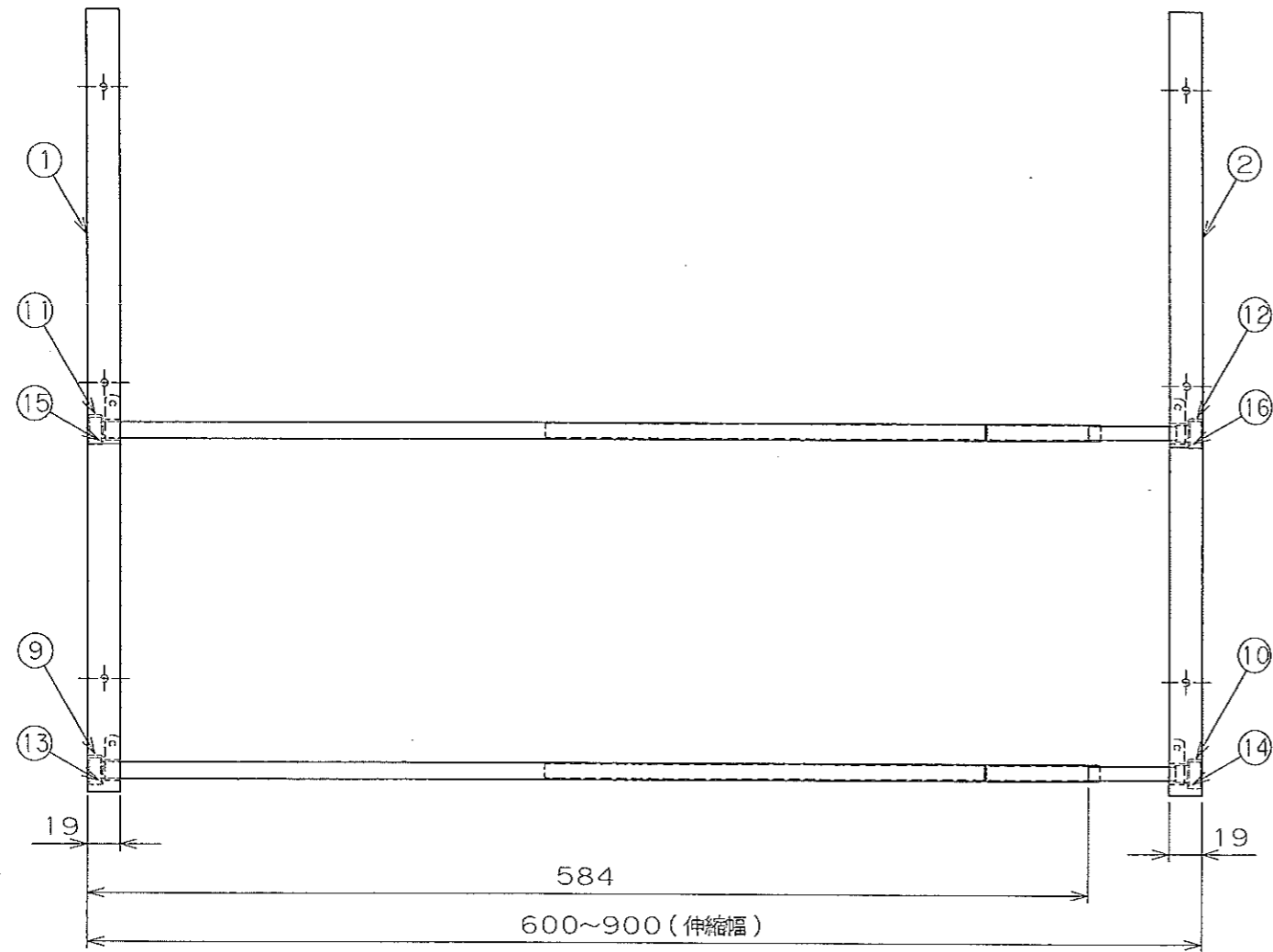
正面図
